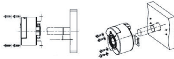
Figura 7 - Encoder ad albero cavo
