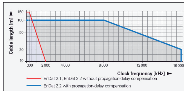
Figura 16 - EnDat 2.1, EnDat 2.2
