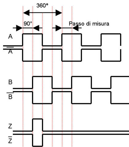
Figura 11 - Segnali incrementali onde quadre TTL
