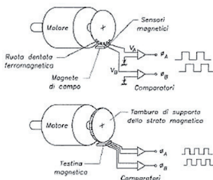
Figura 2 - Sistemi a riluttanza e a banda magnetica
